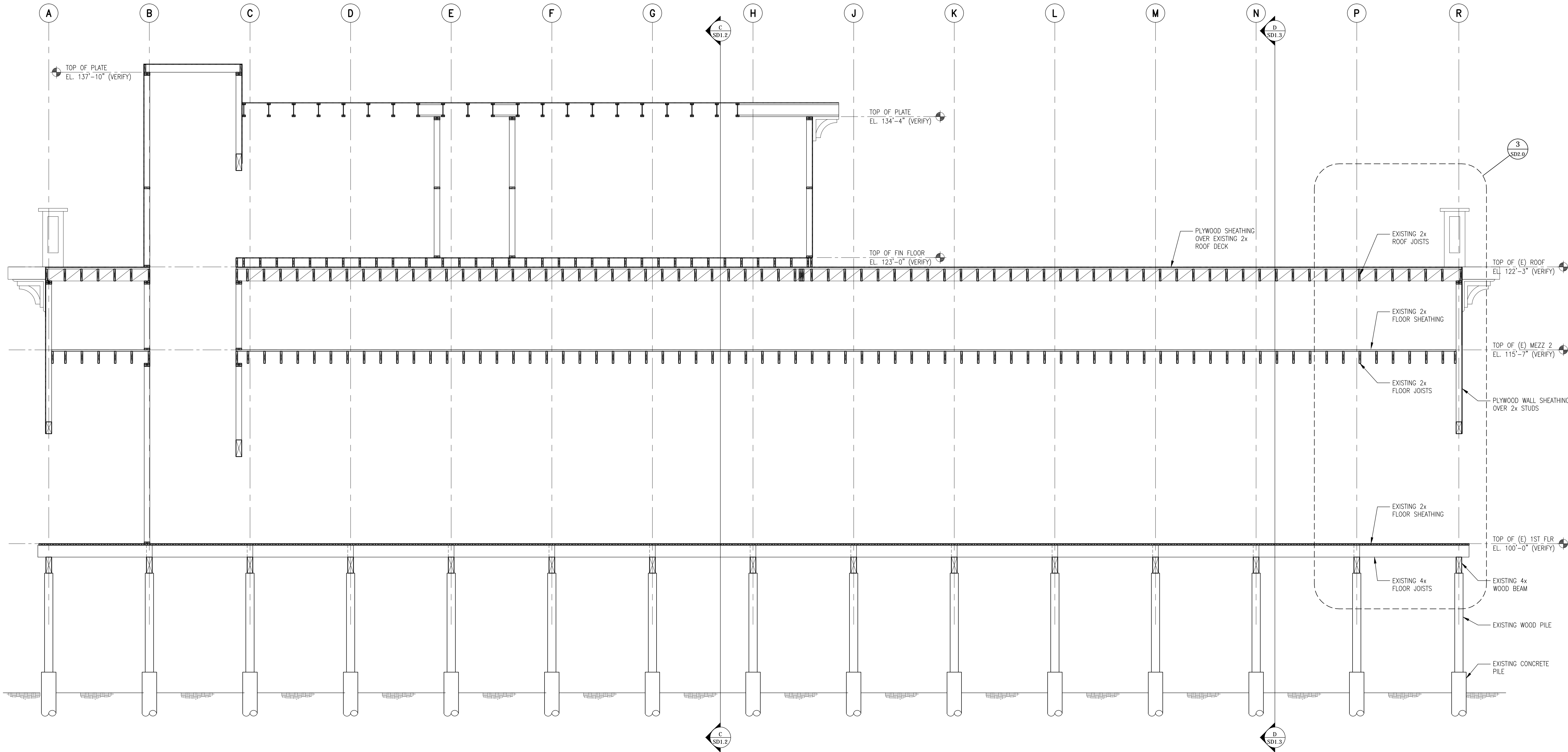
SECTION A-A
